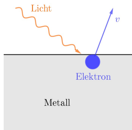
Der Fotoeffekt: Licht kann ein Elektron aus einer Metalloberfläche heraus schlagen
